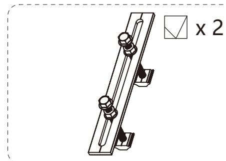
Bottom fasteners Aluminium-Klemmplatte für Geländer
